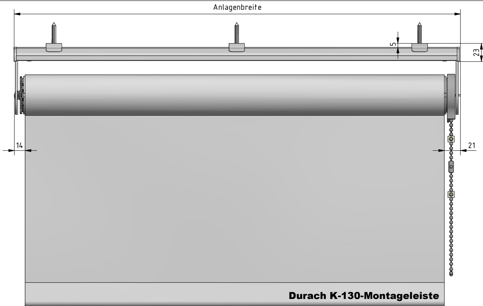
Montage: Montageleiste mit Montageclip
