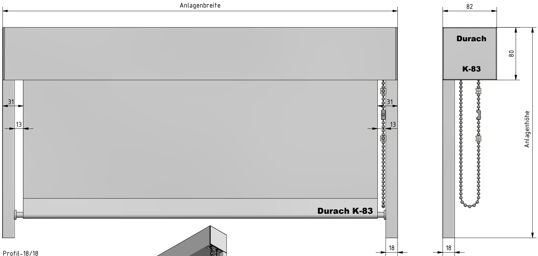
Profil-18/18 Maßstab ( 1 : 1 )
