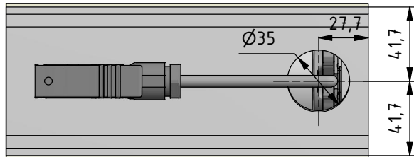
Ansicht von oben Kabelführung Hirschmannstecker
