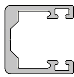
SF-18/18 Maßstab (1 : 1)
