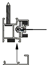
Seitenführung 34/36: 2-tlg. mit Führungsschiene, ZIP-Behang und Einlauftrichter
