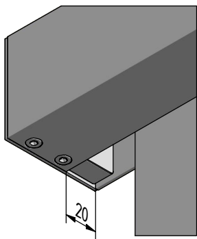
Detail A Stoffauslass
