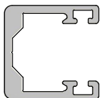
Profil-18/18 Maßstab ( 1 : 1 )
