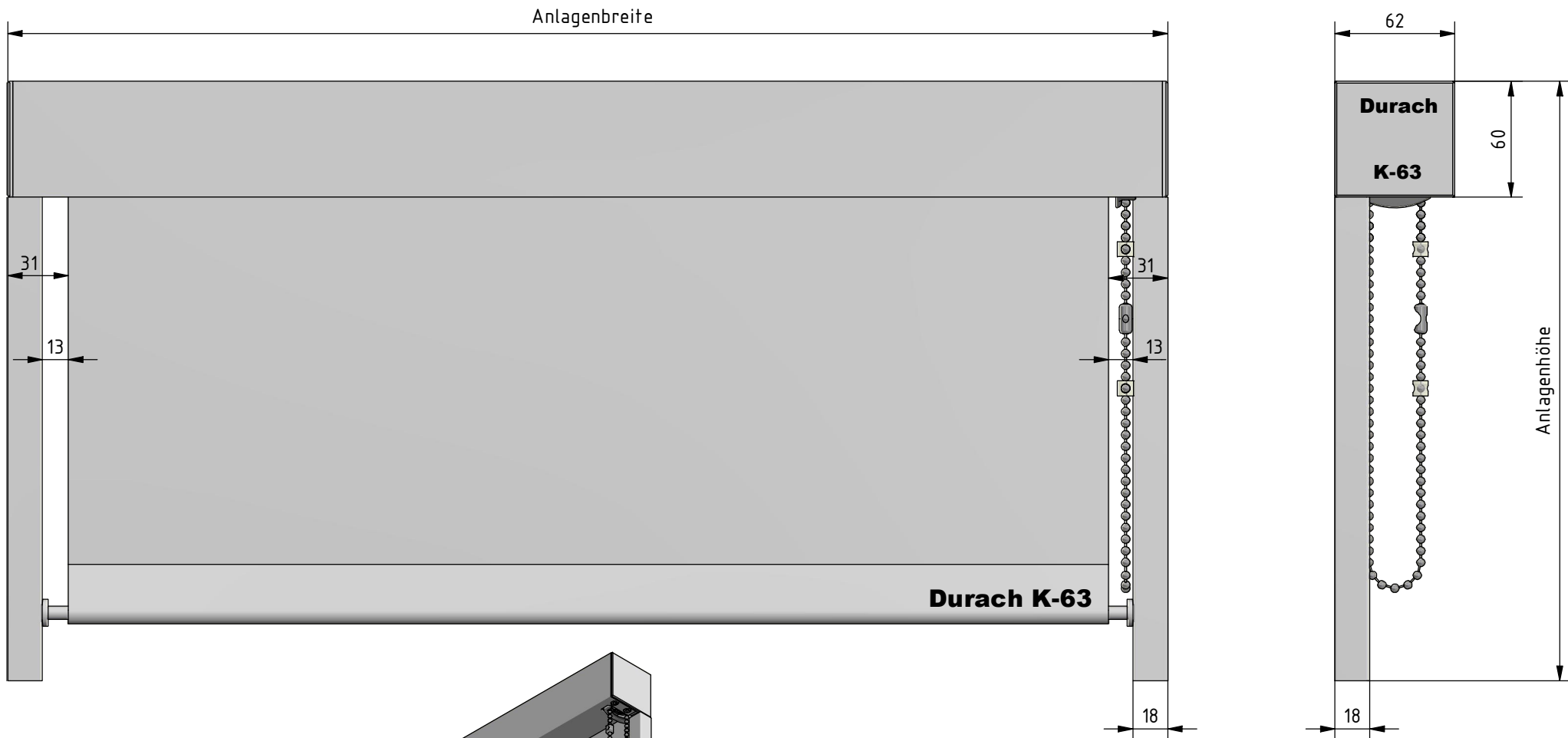
Profil-18/18 Maßstab ( 1 : 1 )
