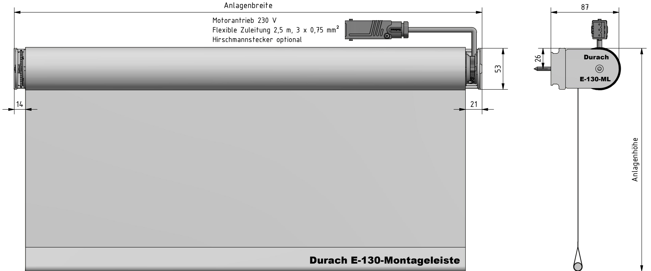
Montage: Montageleiste mit Durchgangsbohrungen
