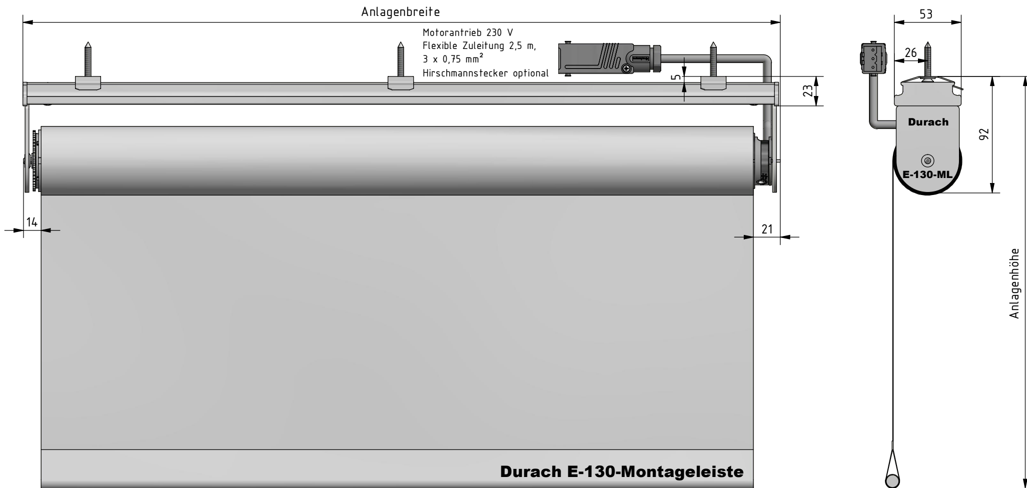
Montage: Montageleiste mit Montageclip
