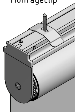
Montage: Montageleiste mit Montageclip
