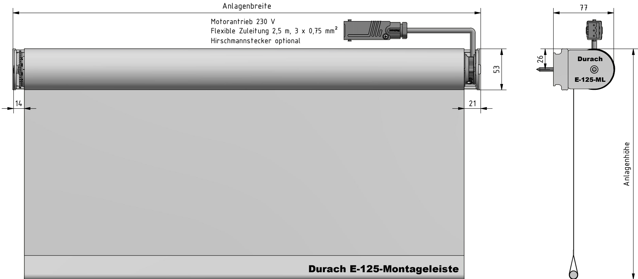
Montage: Montageleiste mit Durchgangsbohrungen
