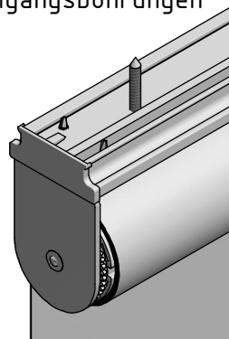
Montage: Montageleiste mit Durchgangsbohrungen
