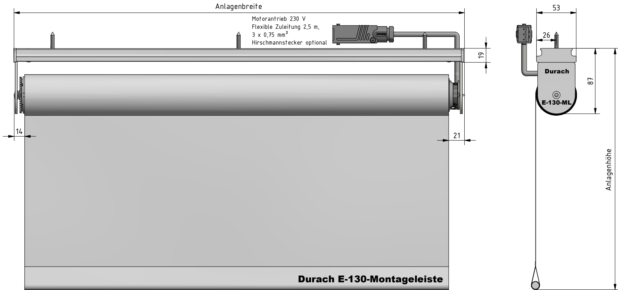
Montage: Montageleiste mit Durchgangsbohrungen
