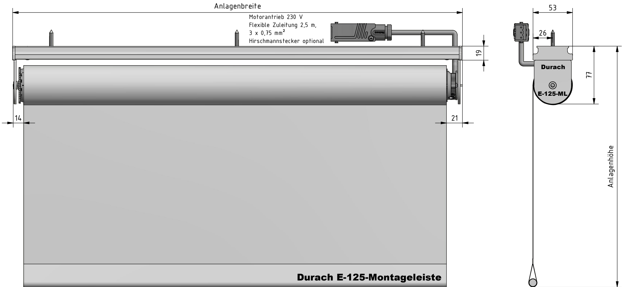
Montage: Montageleiste mit Durchgangsbohrungen
