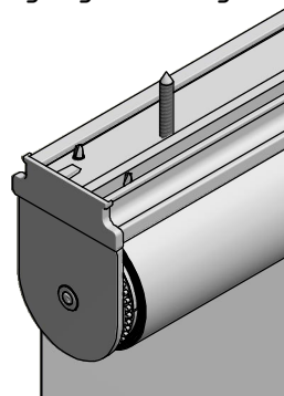
Montage: Montageleiste mit Durchgangsbohrungen
