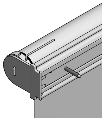
Montage: Montageleiste mit Durchgangsbohrungen
