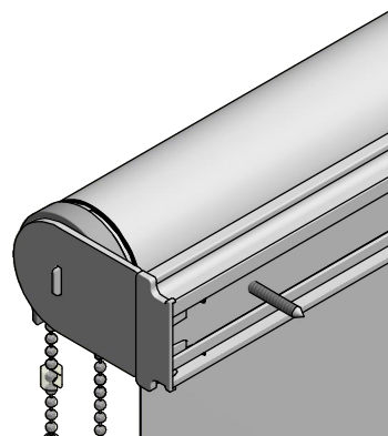
Montage: Montageleiste mit Durchgangsbohrungen
