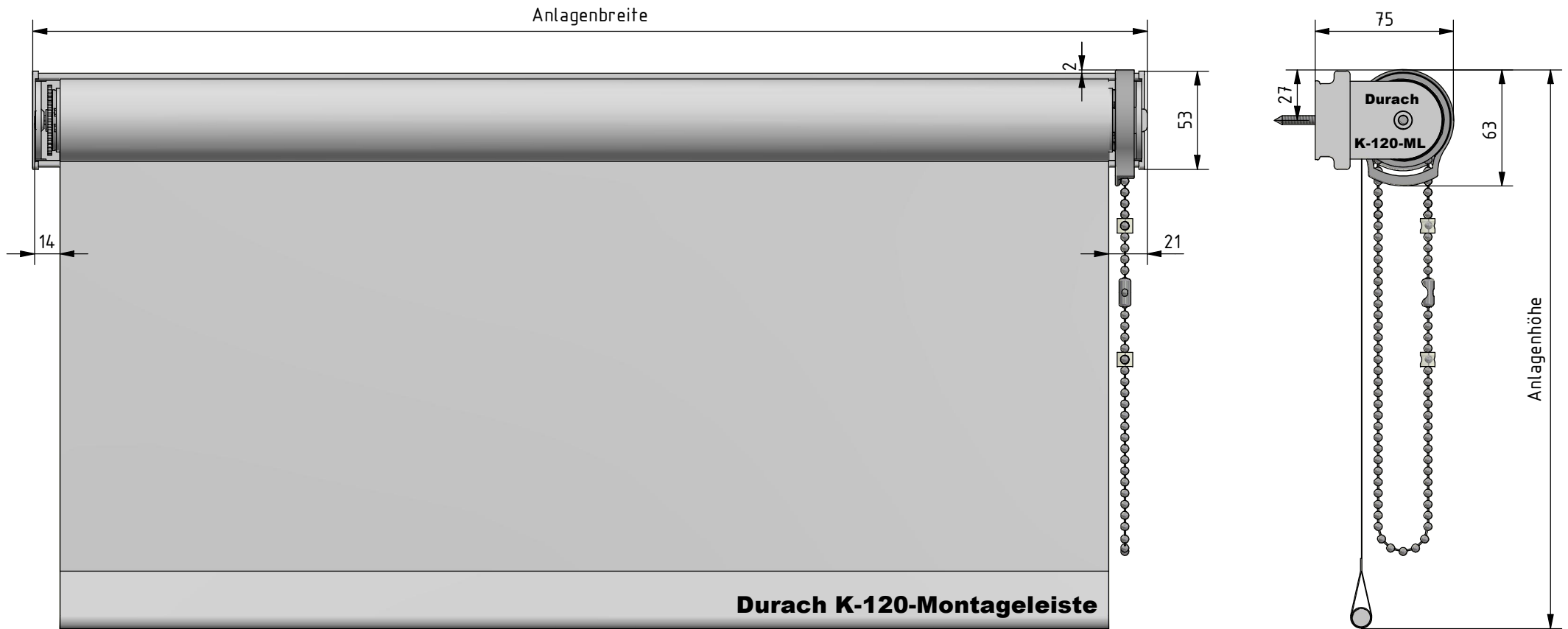
Montage: Montageleiste mit Durchgangsbohrungen
