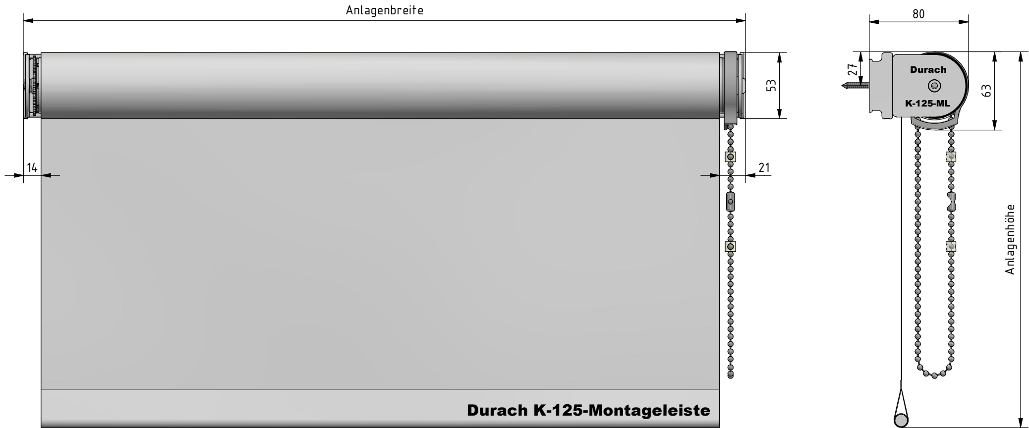
Montage: Montageleiste mit Durchgangsbohrungen
