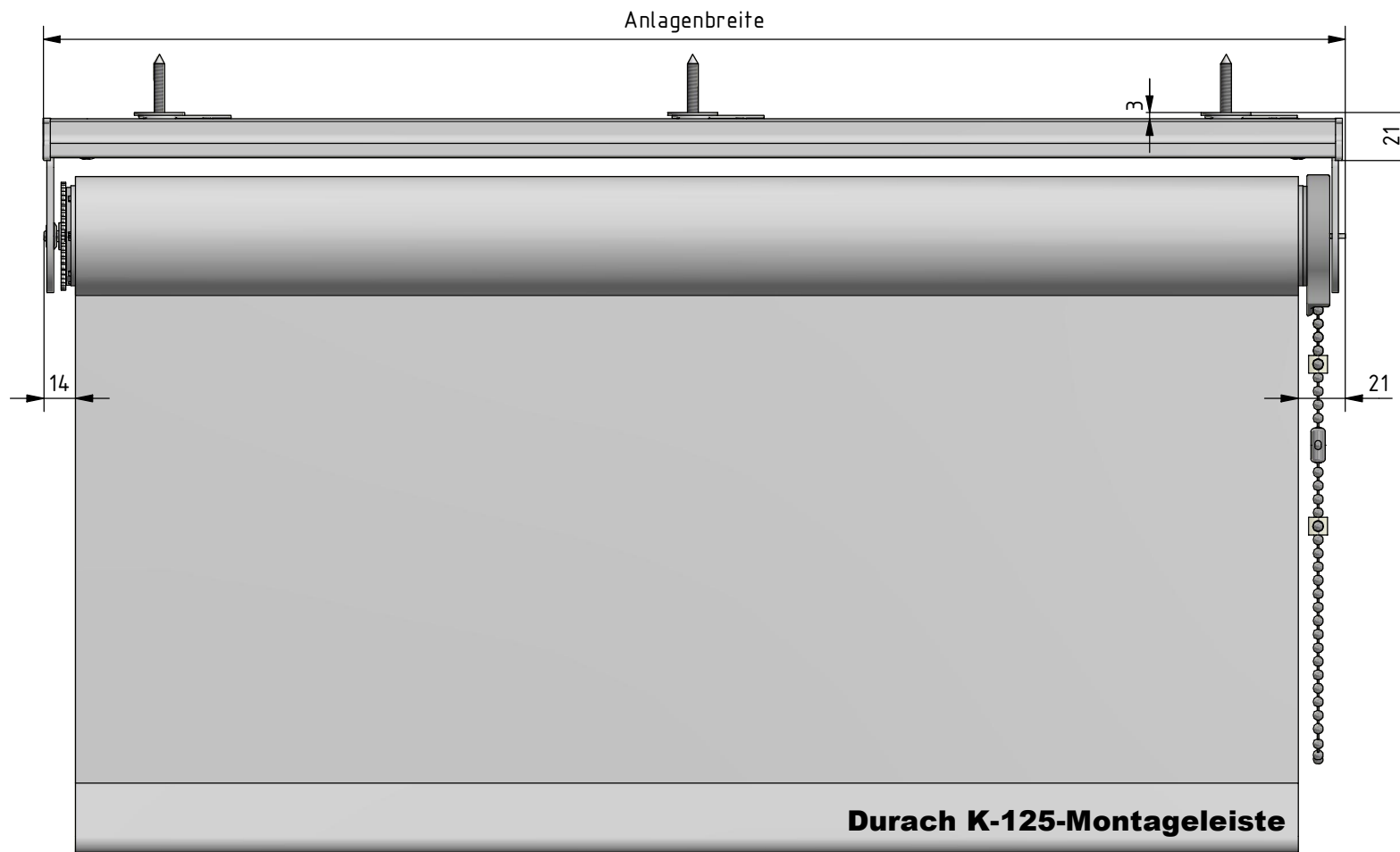
Montage: Montageleiste mit Schnellspanner
