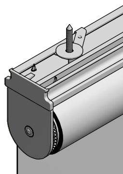
Montage: Montageleiste mit Schnellspanner
