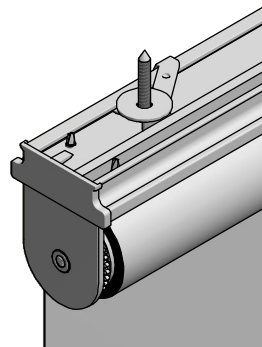
Montage: Montageleiste mit Schnellspanner
