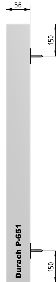
Ansicht vertikal
