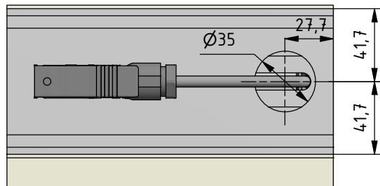
Ansicht von oben Kabelführung Hirschmannstecker
