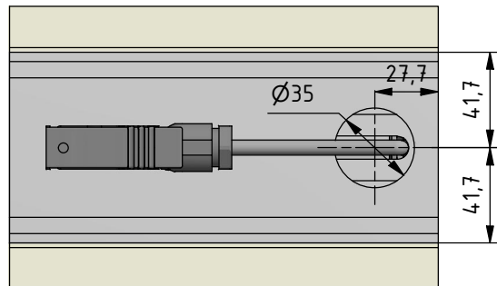
Ansicht von oben Kabelauslass Hirschmannstecker
