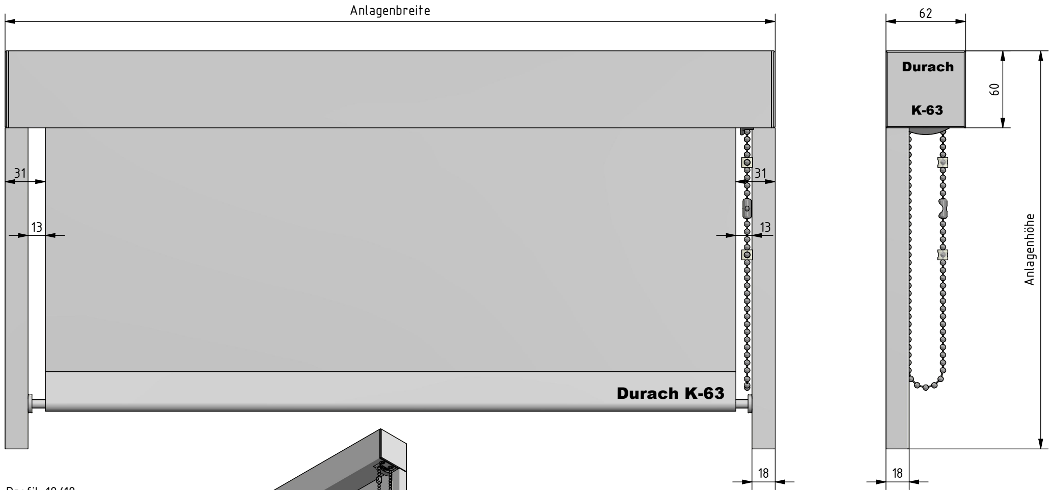
Profil-18/18 Maßstab ( 1 : 1 )
