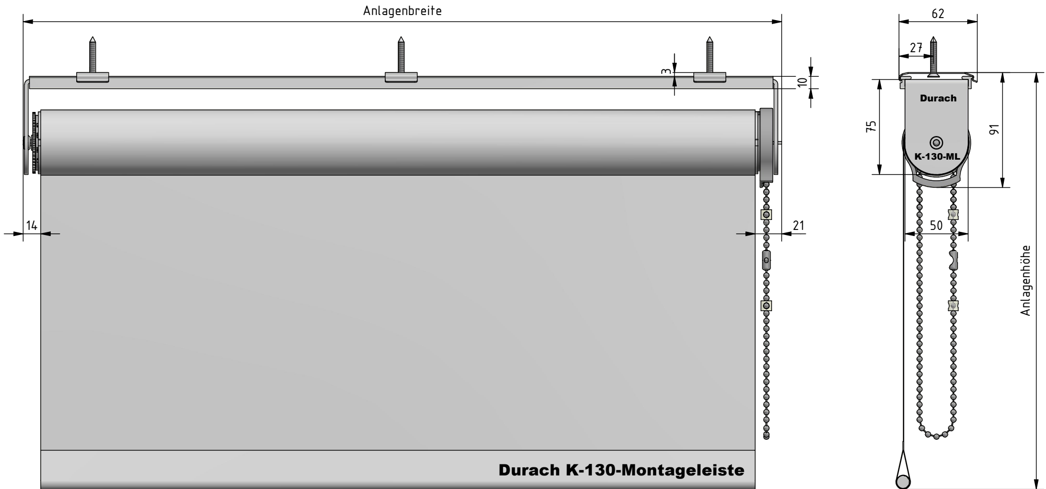
Montage: Montageleiste mit Montageclip
