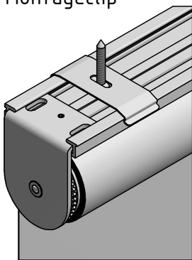
Montage: Montageleiste mit Montageclip
