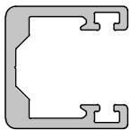
SF-18/18 Maßstab (1 : 1)
