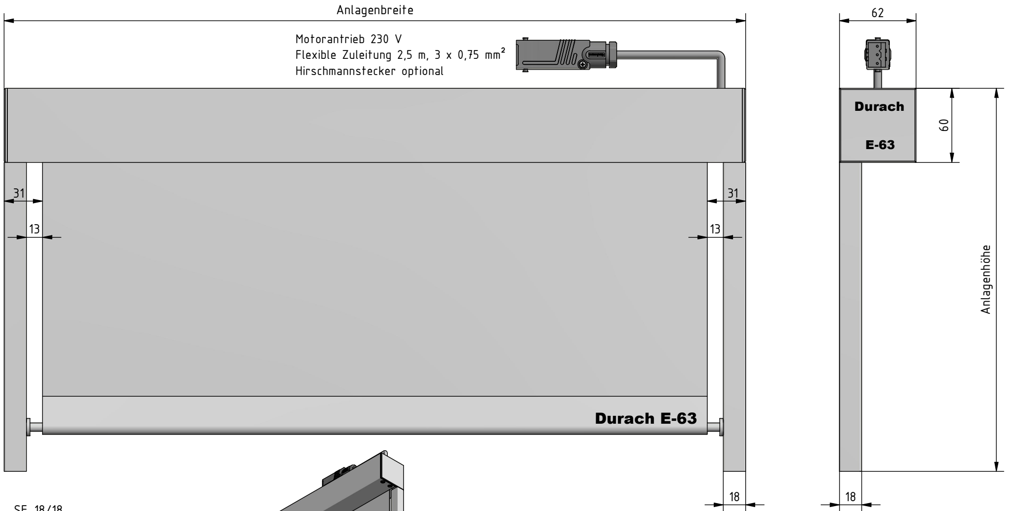
SF-18/18 Maßstab (1 : 1)
