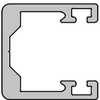
SF-18/18 Maßstab (1 : 1)
