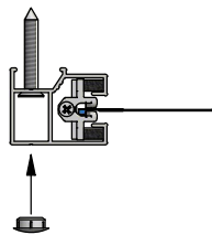
Seitenführung 28/35: 2-tlg. mit Führungsschiene, ZIP-Behang und Einlauftrichter
