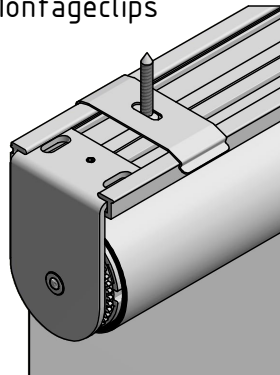
Montage: Montageleiste mit Montageclips
