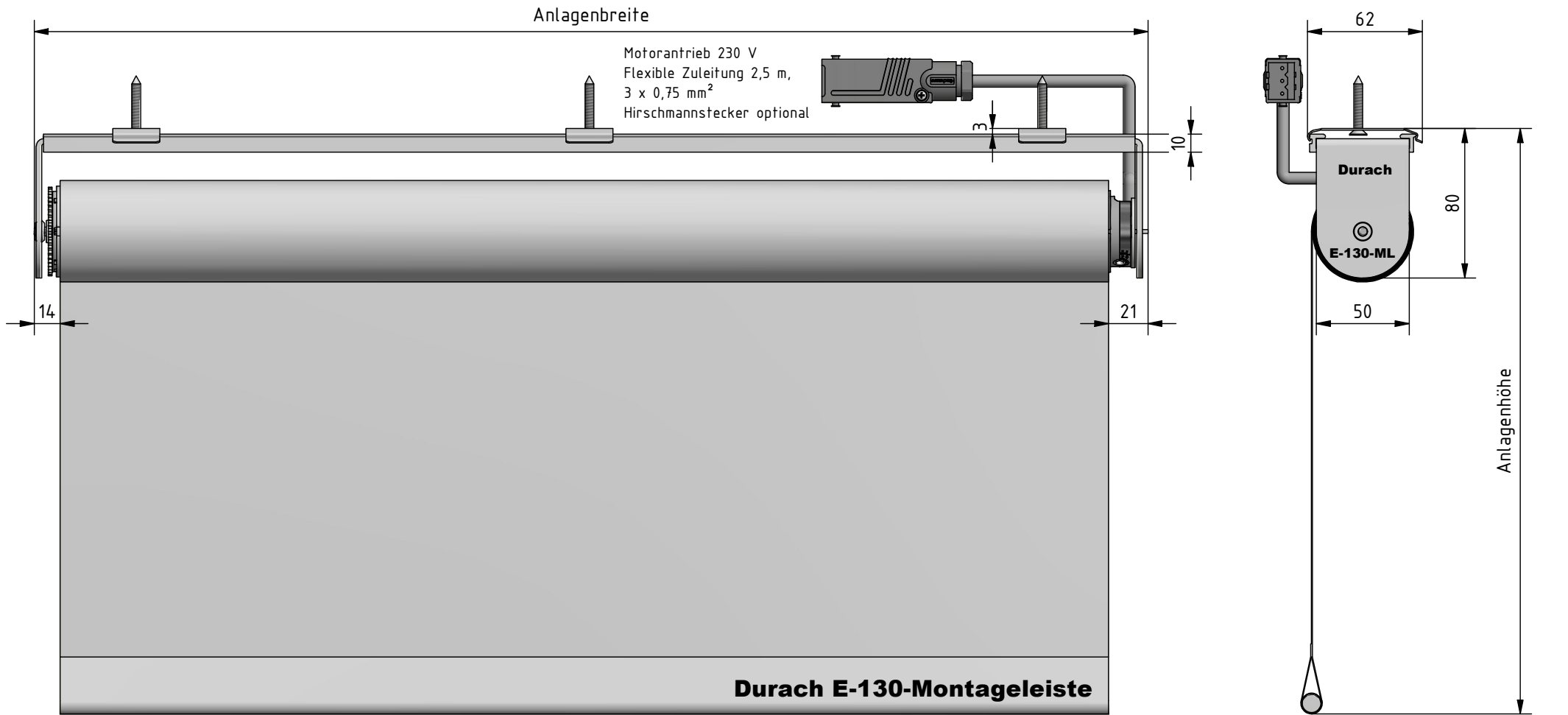
Montage: Montageleiste mit Montageclips
