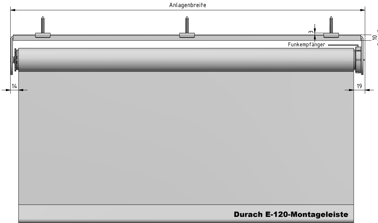
Montage: Montageleiste mit Montageclips
