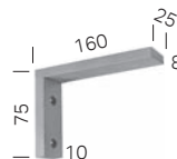
Wandträger 16 cm
