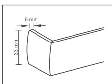
Holzblende mit Ecke 6 mm 33 mm Aufpreis 15,50 €
