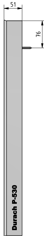
Ansicht vertikal
