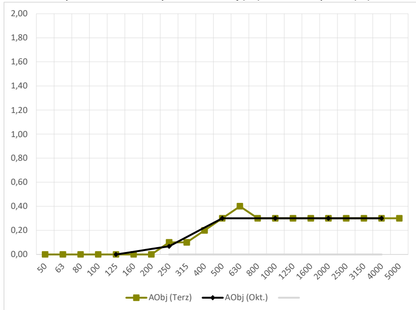
Äquivalente Schallabsorptionsfläche A Obj (m 2 ) über der Frequenz F (Hz)
