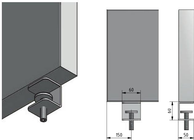
Tischhalter
