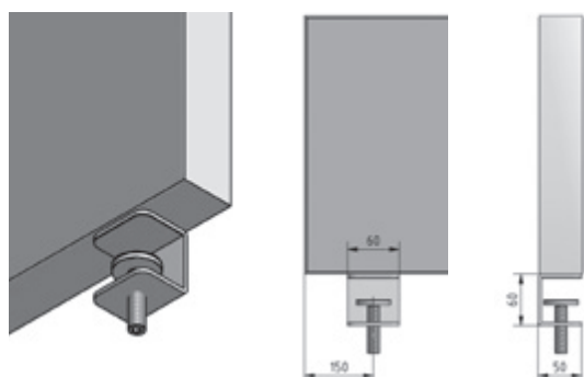
Standfuß flach (Mehrpreis) Art. Nr. P-5040
