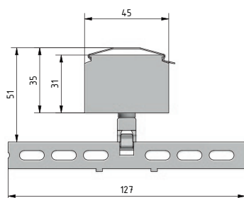
Decke mit Montageclip
