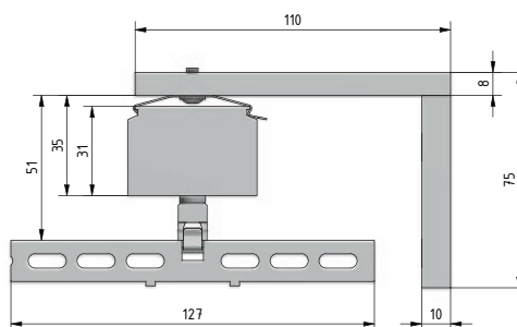
Montage mit Wandträger
