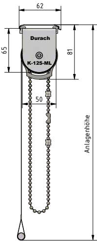
Deckenmontage
