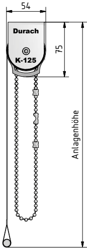
Deckenmontage
