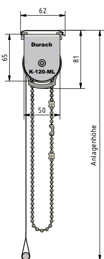
Deckenmontage
