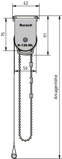
Deckenmontage
