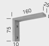
Wandträger 16 cm
