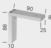
Wandträger 9 cm
