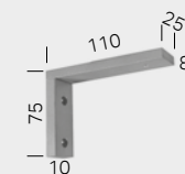
Wandträger 11 cm
