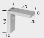
Wandträger 7 cm
