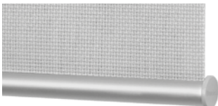
Beschwerungsstab außenliegend rund Aluminium, Ø 16 mm Art.-Nr. R-1292
