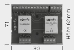
4-fach Trennrelais TR4
