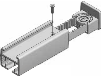
Umlenkung Glydea „Mini“
