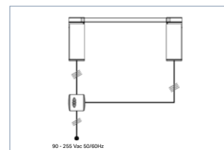
P-595-Tandem
