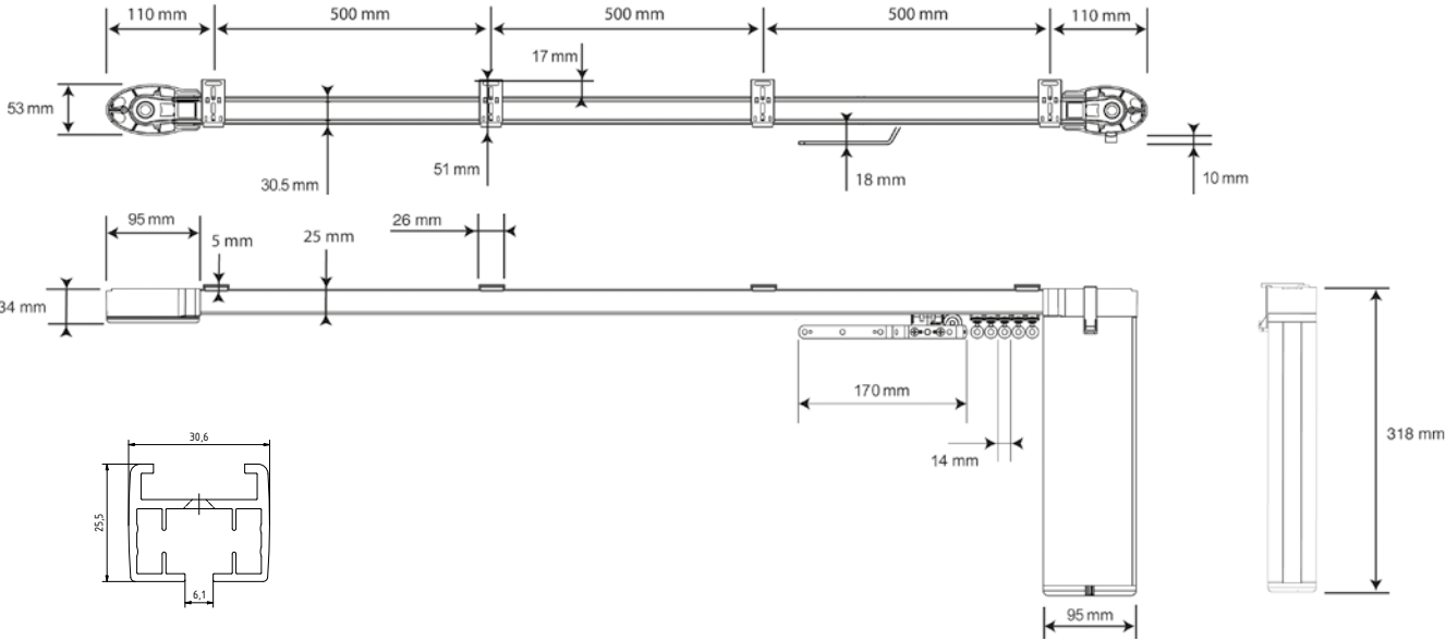
Umlenkung Glydea „Mini“
