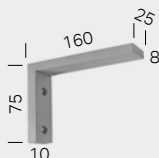
Wandträger 16 cm
