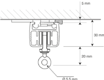
Montage mit Deckenclip
