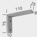
Wandträger 11 cm
