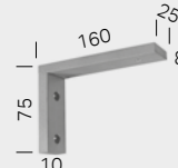
Wandträger 16 cm
