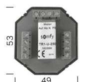
1-fach Trennrelais TR1
