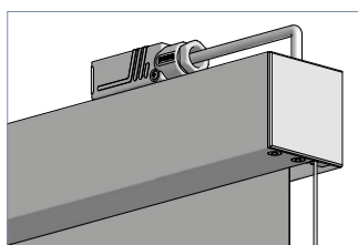
E-66 Seilverspannung
