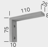
Wandträger 11 cm
