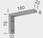
Wandträger 16 cm
