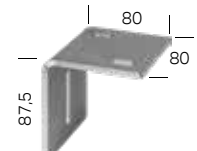
Montagewinkel für MP-80
