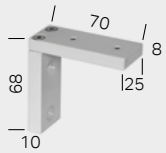
Wandträger 7 cm
