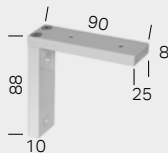
Wandträger 9 cm
