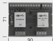
4-fach Trennrelais TR4
