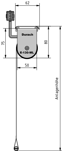
Deckenmontage
