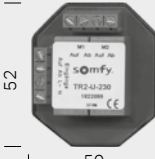
2-fach Trennrelais TR2
