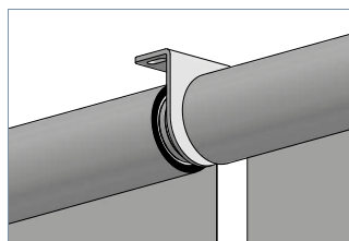
E-125-K Kopplungsträger*
