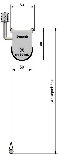
Deckenmontage
