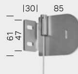
Träger Seilverspannung E-130
