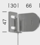
Träger Seilverspannung E-120
