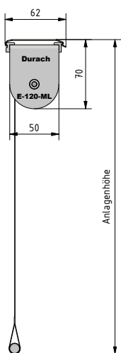
Deckenmontage
