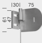
Träger Seilverspannung E-125
