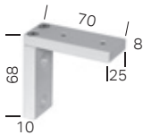
Wandträger 7 cm
