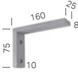
Wandträger 16 cm
