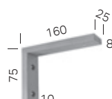
Wandträger 16 cm
