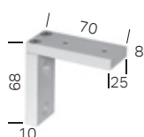
Wandträger 7 cm
