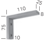
Wandträger 11 cm
