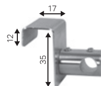
Halter 2 cm durchgehend zum Einhängen am Fenster- rahmen (Rahmenstärke: 17 mm)
