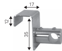
Halter 2 cm durchgehend zum Einhängen am Fenster- rahmen (Rahmenstärke: 17 mm)
