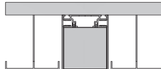
Einbau in abgehängte Decke aus Metall (MP-80-V2)
