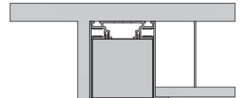
Einbau in abgehängte Decke Wand-/ Fassadenbündig (MP-80-V3)
