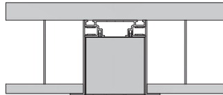
Einbau in abgehängte Decke (MP-80-V1)
