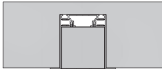
Einbau in Decke (MP-80-V1)
