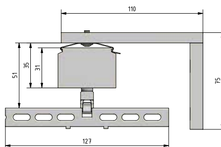
Montage mit Wandträger
