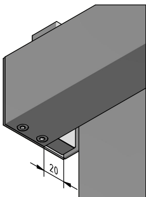
Detail A Stoffauslass
